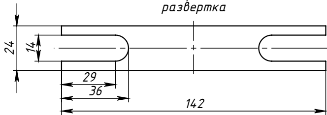
Поз.5 (Прокладка) развертка
