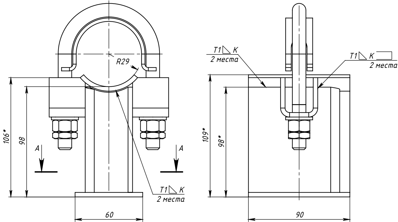
Поз.6 (Хомут)
