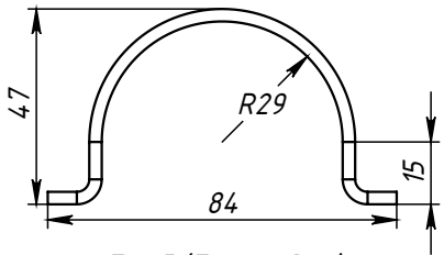
Поз.5 (Прокладка) развертка
