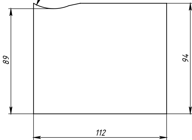
Поз.2 (Угольник) развертка
