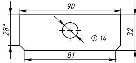
Поз.4 (Ушко) развертка
